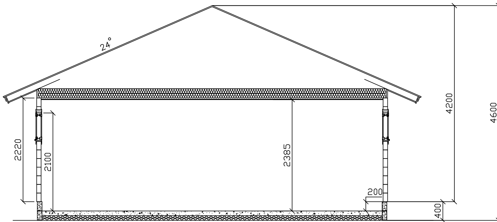
LEIKKAUS A-A
