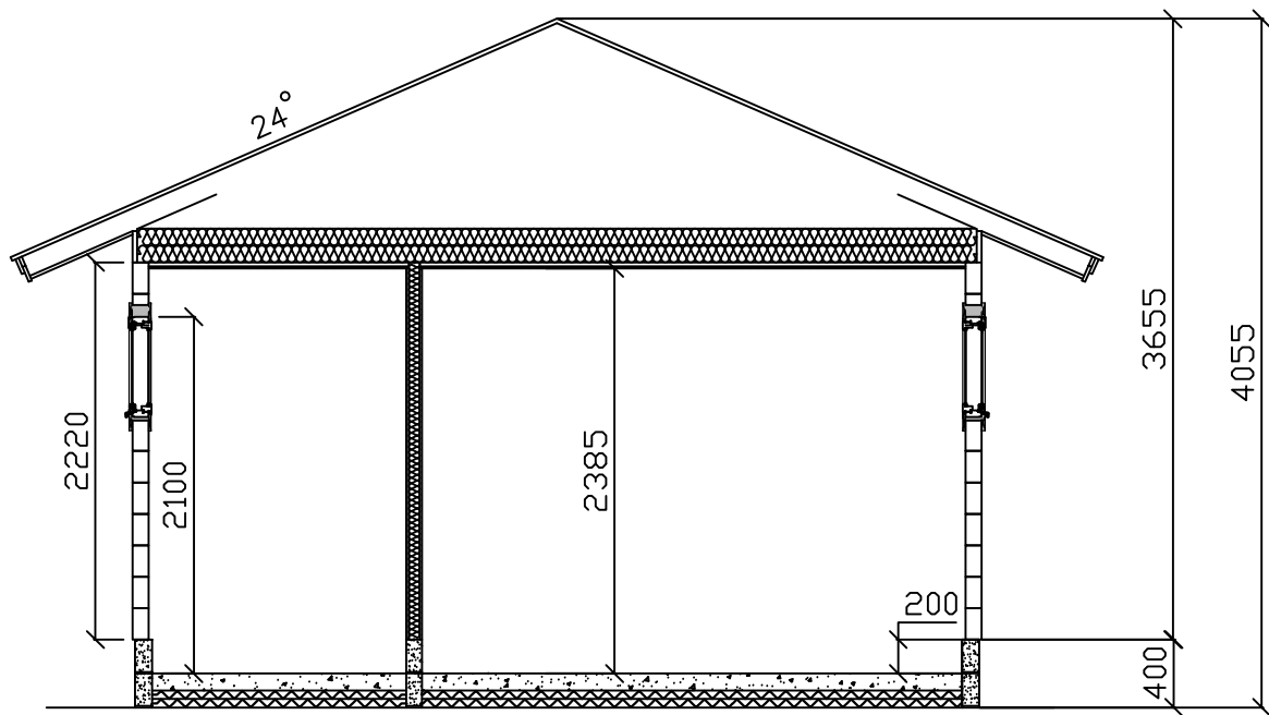
LEIKKAUS A-A
