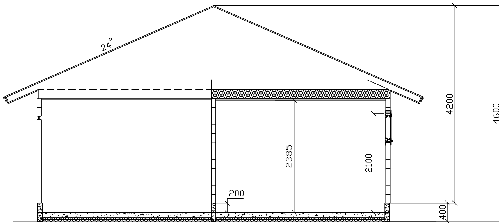
LEIKKAUS A-A
