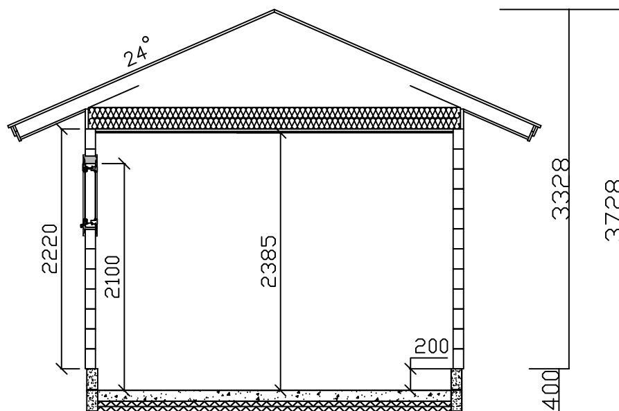
LEIKKAUS A-A
